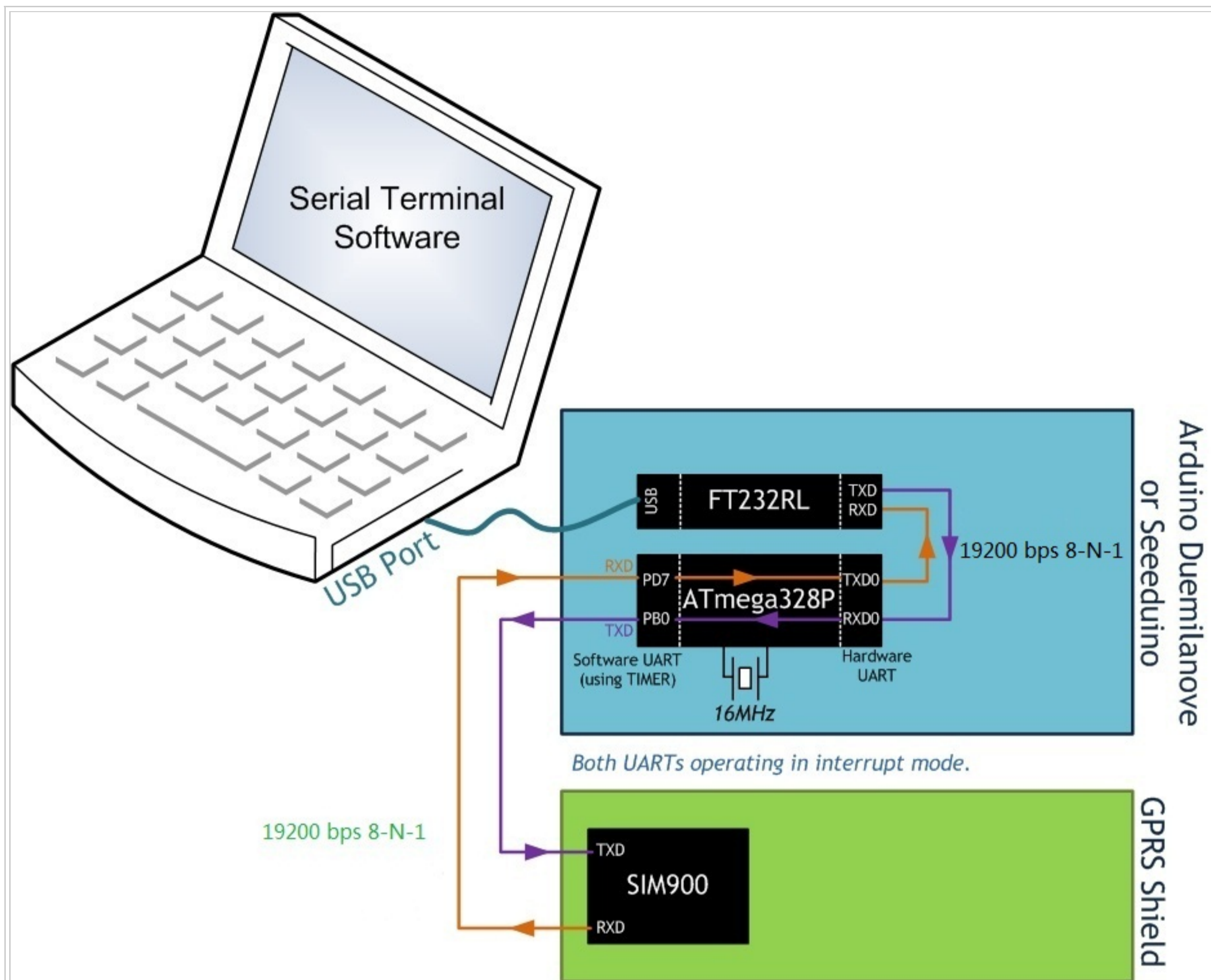
GPRS arduino uart.jpg
